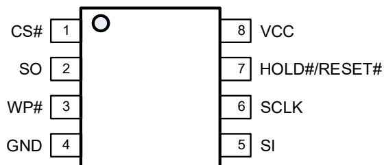
8-Lead SOP(208mil)
